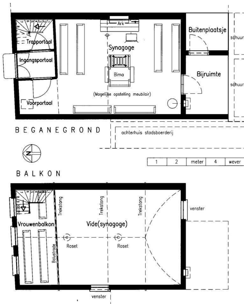
(9) Reconstructietekening van de stichtingsfase met de situaties van de begane grond en het vrouwenbalkon. (Tekening G.J. Wever)
