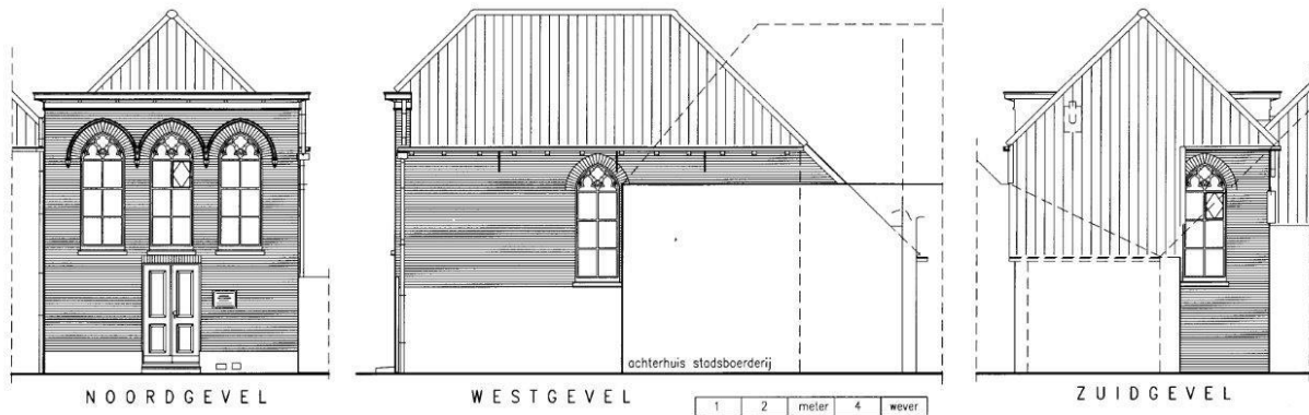
(6) Reconstructietekening van de gevelbeelden uit de stichtingsfase. De missende oostgevel is grotendeels afgedekt met het buurpand en daarom niet zelfstandig weergegeven. Voor de westgevel staan de gestippelde contouren van de stadsboerderij (perceel 83). Voor de zuidgevel staan de gestippelde contouren van de achterliggende stadsboerderij (perceel 86) (Tekening G.J. Wever)
